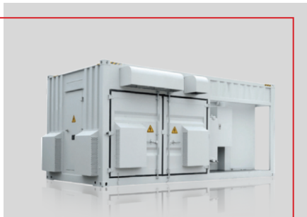
YBW F/G-40.5/0.69 户外预装式变电站 (风电 / 光伏专用)
